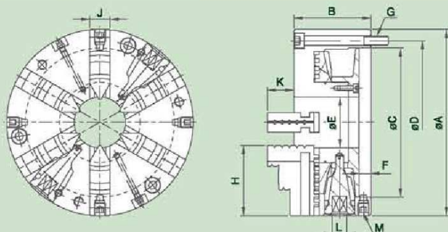
尺寸圖 > Dimensions
