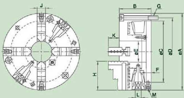
尺寸圖 > Dimensions
