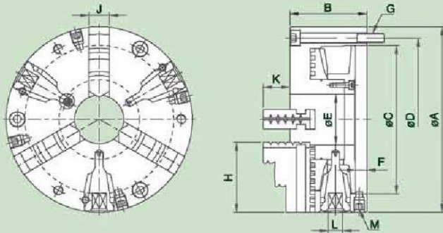
尺寸圖 > Dimensions
